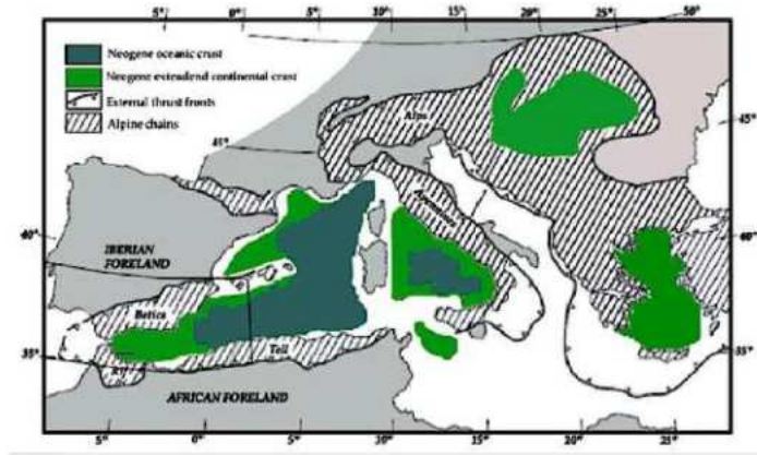
Figure 1 : processus tectonique de rupture de l'axe d'une chaîne poly-orogénique (Varisque et Alpine) lors de l'ouverture d'un bassin océanique
