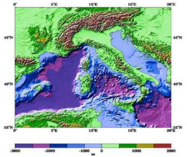
Figure 2 : exemple unique de fracturation d'une chaîne de montagnes poly-orogénique
